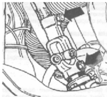
Рис. 3.40 Снятие хомута рулевого управления. Стелками показаны крепежные гайки
