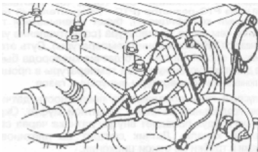
Рис. 5.67 Расположение датчика распредвала — Volvo-960
