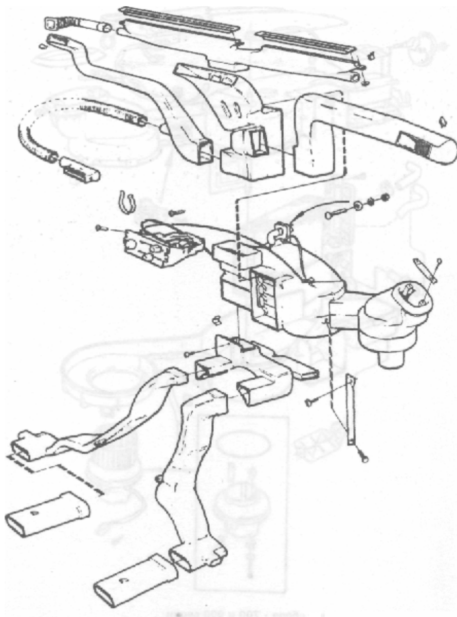
Рис. 6.7 Стандартный обогреватель 700 и 900 серий
