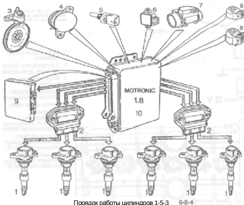
Рис. 2. 37 Основные компоненты управления зажиганием в автомобиле Volvo 960. Обратите внимание на установленные на свечах индивидуальные катушки зажигания
