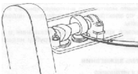
Рис. 2.45 Проверка зазоров клапанов, цилиндр N 1 двигателя B230F и B230FT
