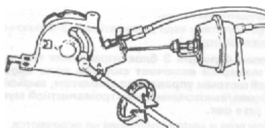
Рис. 5.116 Регулировка тяги воздушной заслонки
