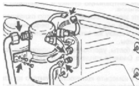
Рис. 6.20 Снятие ресивера/осушителя
