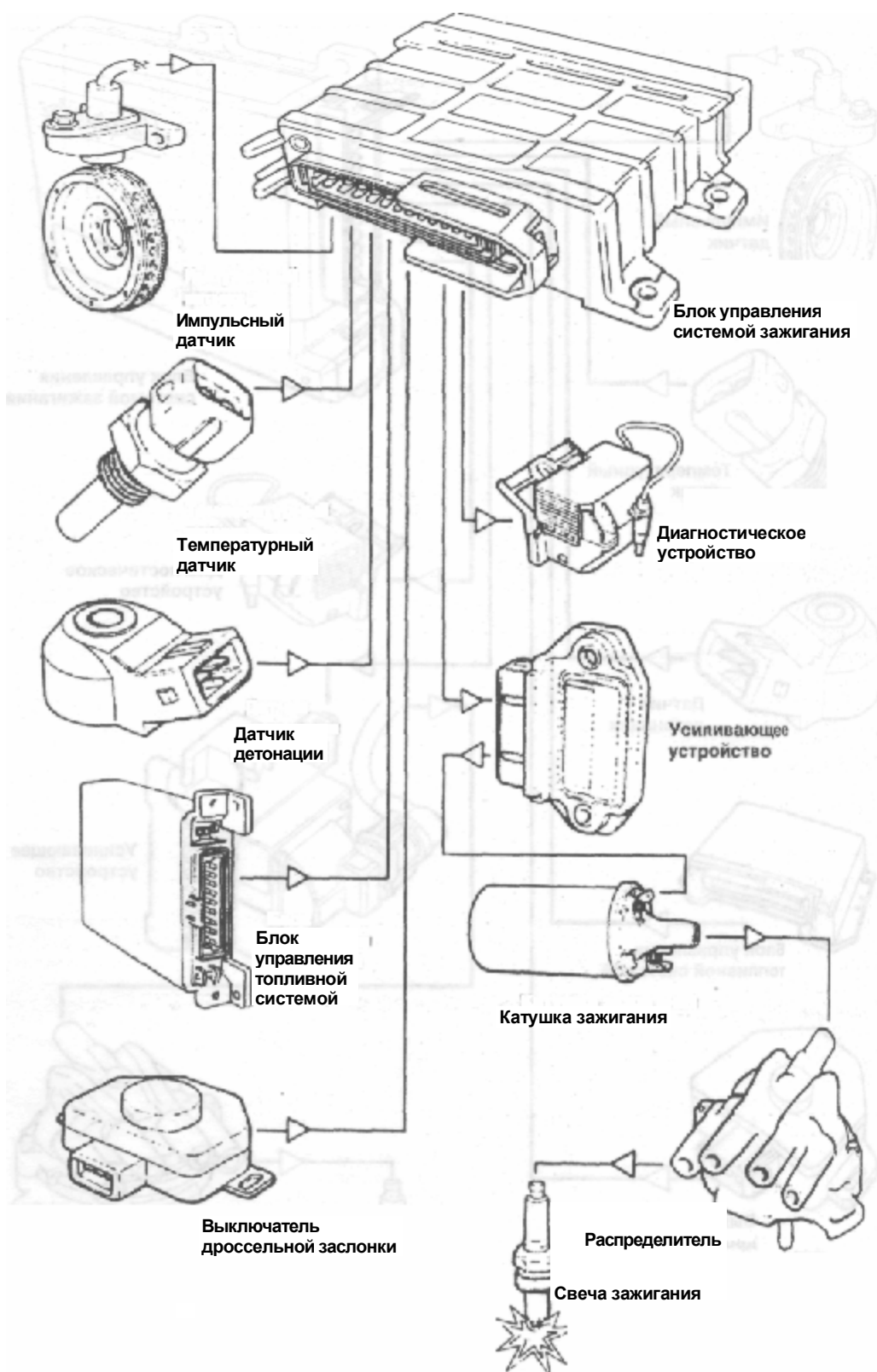
Рис. 2.9 Блок-схема системы зажигания EZ116K
