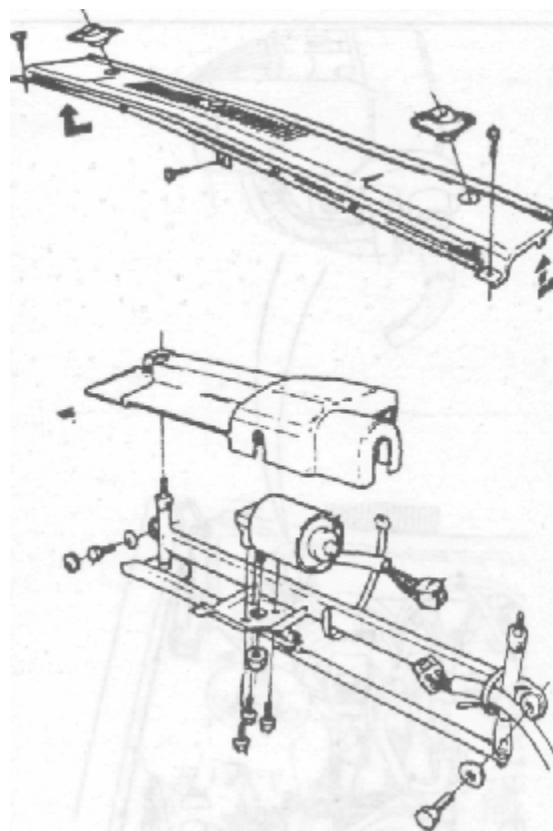
Рис. 6.31 Снятие малого капота и узла привода в сборе — 700 Серия
