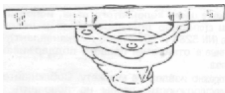
Рис. 3.49 Проверка места разъема масляного насоса на плоскостность — Двигатель B234F
