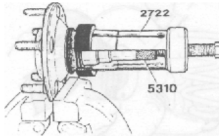
Рис. 7.44 Снятие внутреннего кольца со ступицы независимая подвеска
