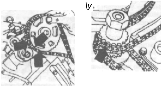
Рис. 3.63 Последовательность установки цепи привода правого распределительного вала - Двигатель B280F
