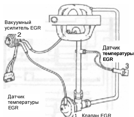
Рис. 5.45 Компоненты системы EGR
