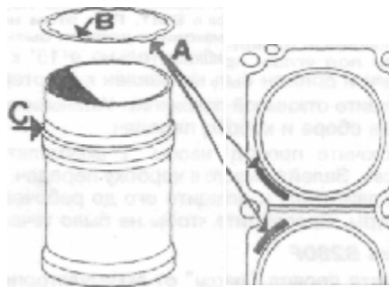
Рис. 3.73 Правильное расположение кольца гильзы цилиндра — Двигатель B280F
