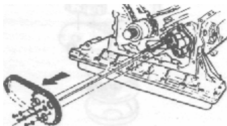
Рис. 3.46 Снятие звездочки и цепи масляного насоса - Двигатель B280F
