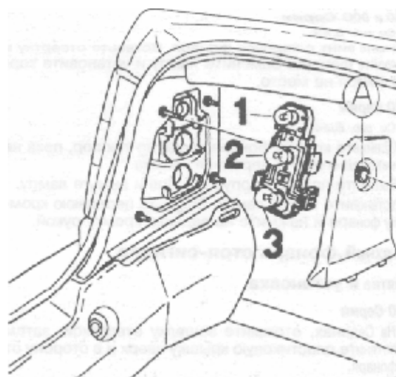
Рис. 6.41 Замена ламп заднего фонаря — показано для Седана 740 и 900 Сери
