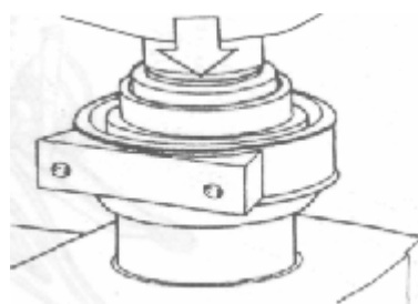
Рис. 7.36 Установка подшипника в сепаратор. Вверху и внизу показан применяемый инструмент
