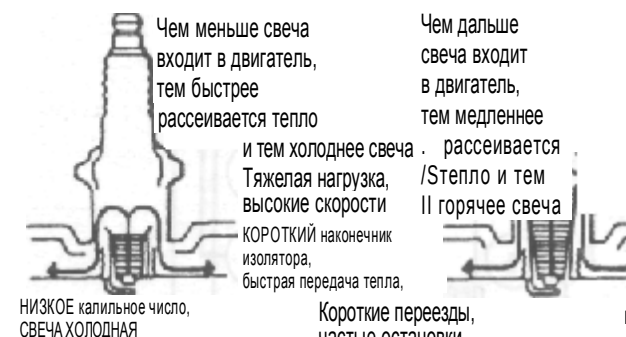
Рис. 2.2 Калильное число
