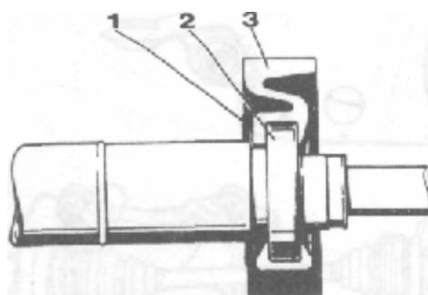
Рис. 7.35 Правильная установка подшипника в резиновой опоре 1. Пылезащитный колпак, 2. Подшипник, 3. Резиновая опора
