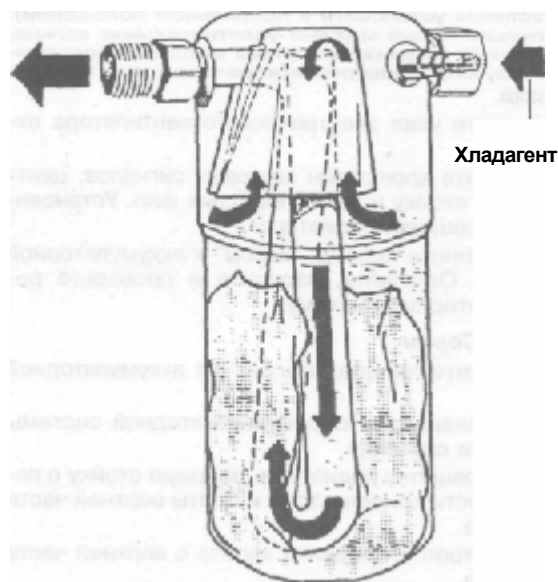
Рис. 6.21 Работа ресивера/осушителя
