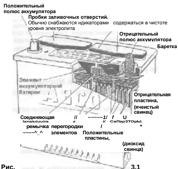
Рис. 3.1 Аккумуляторная батарея
