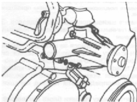
Рис. 3.24 Установка водяного насоса — Двигатель B230F
