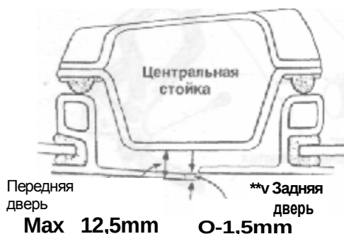
Рис. 10.1 Убедитесь, что зазор между центральной стойкой и внешней стороной передней двери не превышает 12,5 мм. Задняя дверь должна отстоять на 10,5 мм. — Показана серия 700, на остальных — аналогично.
