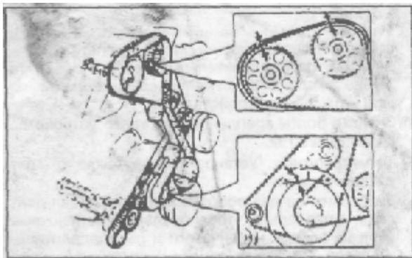
Рис. 3.57 Совмещение установочных меток — Двигатель B234F
