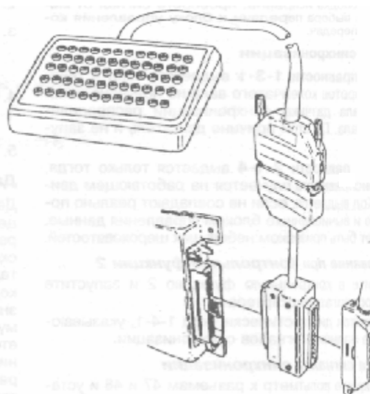
Рис. 2.42 Расположение электронного блока управления (ECU) и рекомендуемая предохранительная коробка, используемая для проверки его систем — Volvo-960
