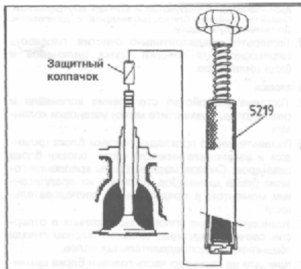
Рис. 3.37 При установке маслоотражательных колпачков всегда ставьте защитные колпачки — Двигатель B230F
