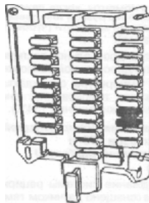
Рис. 5.72 Предохранители N30 и 31 топливного насоса
