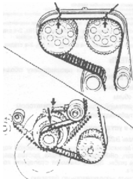
Рис. 3.14 Метки на приводном ремне должны совместиться с меткой на шкиве. Вначале устанавливайте ремень на правый шкив - двигатель B234F
