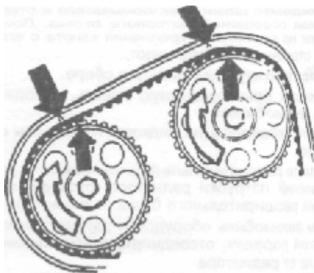
Рис. 3.15 Правильное положение шкивов распредвалов перед затяжкой регулировочного шкива
