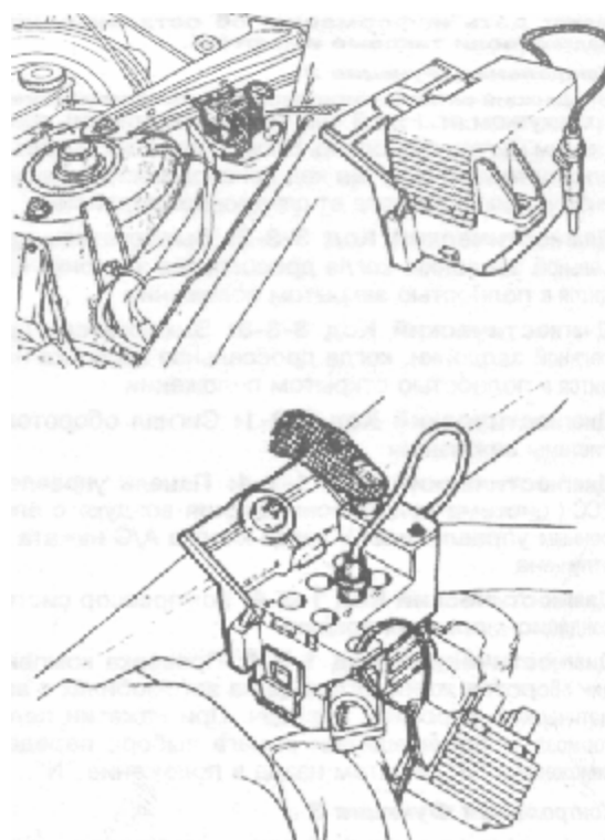
Рис. 5.28 Считывание кодов неисправностей топливной системы Volvo
