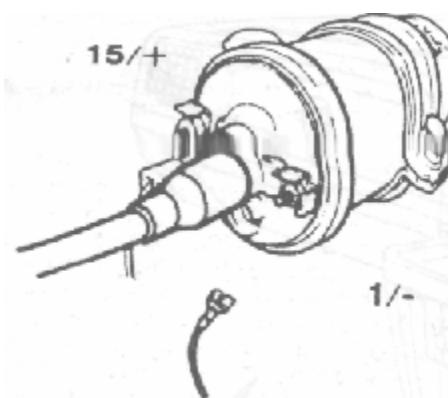
Рис. 5.7 Отсоединение катушки зажигания при проверке компрессии двигателя LH-Jetronic
