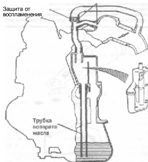
Рис. 1.11 Принудительная вентиляция картера -- двигатель B230F
