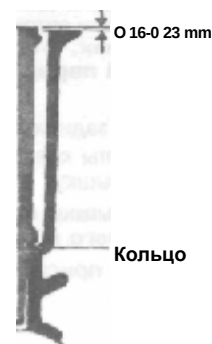
Рис. 3.74 Взаиморасположение гильзы цилиндра, кольца и блока цилиндров — Двигатель B280F
