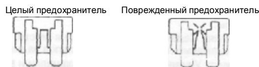
Рис. 6.49 Сравнение неисправного предохранителя с исправным
