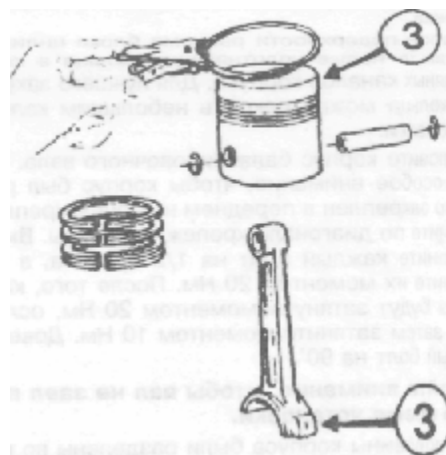
Рис. 3.69 Снятие поршневых колец при помощи специальных плоскогубцев
