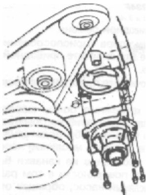
Рис. 3.44 Снятие масляного насоса — Двигатель B234F
