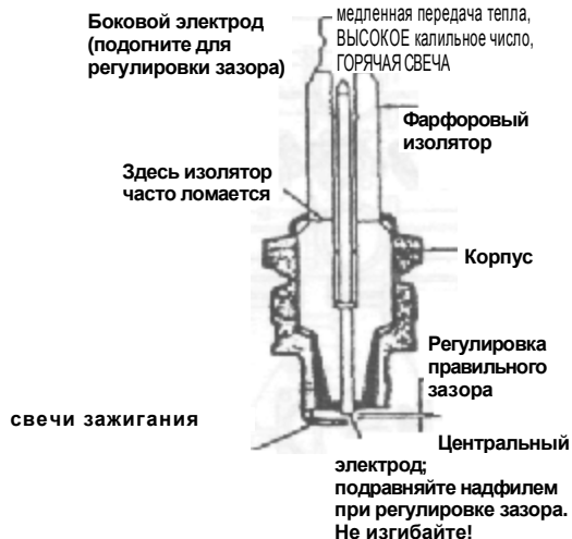
Рис. 2.3 Вид свечи зажигания в разрезе
