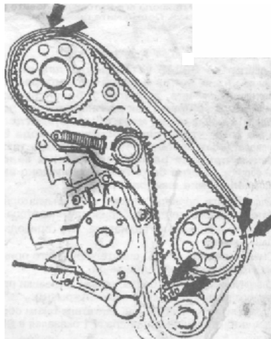
Рис. 3.51 Установка приводного ремня по меткам Двигатель B230F
