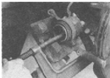
Рис. 9.11 Проталкивание поршней тормозных суппортов в их цилиндрах
