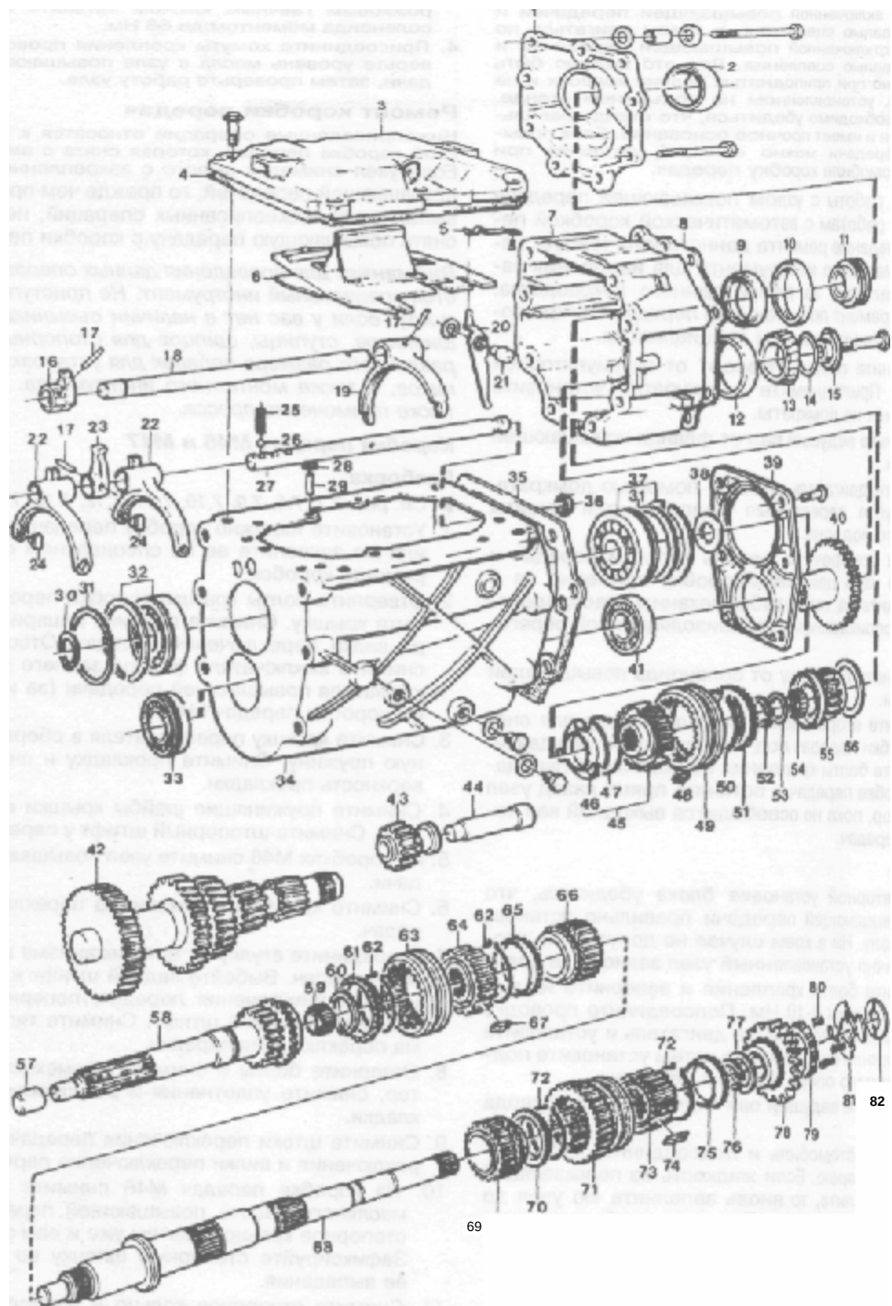
Рис. 7.7 Коробка передач М47 в разобранном виде I. Задняя торцевая крышка, 2. Уплотнение, 3. Верхняя крышка, 4. Прокладка, 5. Пружина, 6. Крышка механизма переключения, 7. Картер пятой передачи, 8. Прокладка, 9. Роликовый подшипник, 10. Внешнее кольцо подшипника, II. Ведущая шестерня спидометра, 12. Внешнее кольцо подшипника, 13. Внутреннее кольцо подшипника, 14. Регулировочная прокладка разной толщины, 15. Шайба, 16. Рычаг поводка штока переключения передач, 17. Штифт, 18. Шток переключения передач, 19. Вилка рычага переключения передач, 20. Рычаг переключения шестерни заднего хода, 21. Ось пальца, 22. Вилка переключения передач, 23. Поводок переключения передач, 24. Упор включения, 25. Пружина, 26. Шарик фиксатора, 27. Шток механизма переключения передач, 28. Пружинная шайба, 29. Направляющий штифт, 30. Стопорное кольцо, 31. Регулировочная прокладка разной толщины, 32. Шариковый подшипник, 33. Роликовый подшипник, 34. Картер коробки передач, 35. Прокладка, 36. Уплотнение, 37. Шариковый подшипник, 38. Регулировочная прокладка разной толщины, 39. Держатель подшипников, 40. Ведущая шестерня, 41. Роликовый подшипник, 42. Промежуточный вал, 43. Зубчатое колесо заднего хода, 44. Вал, 45. Ступица синхронизатора, 46. Ведущий фланец, 47. Пружина, 48. Направляющая шпонка (собачка), 49. Пружина, 51. Кольцо синхронизатора, 52. Стопорное кольцо, 53. Распорная втулка, 54. Игольчатый подшипник, 55. Зубчатое колесо пятой передачи, 56. Распорная втулка, 57. Муфта, 58. Ведущий вал, 59. Игольчатый подшипник, 60. Стопорное кольцо, 61. Кольцо синхронизатора, 62. Пружина, 63. Скользящая муфта, 64. Ступица синхронизатора, 65. Кольцо синхронизатора, 66. Зубчатое колесо третьей передачи, 67. Направляющая шпонка, 68. Вторичный вал, 69. Зубчатое колесо второй передачи, 70. Кольцо синхронизатора, 71. Скользящая муфта, 72. Пружина, 73. Ступица синхронизатора, 74. Направляющая шпонка, 75. Кольца синхронизатора, 76. Стопорное кольцо, 77. Шайба, 78. Зубчатое колесо (шестерня) первой передачи, 79. Конус демпфера, 80. Пружина, 81. Ведущий фланец, 82. Упорная шайба (если она не устанавливается вместе с демпфером)
