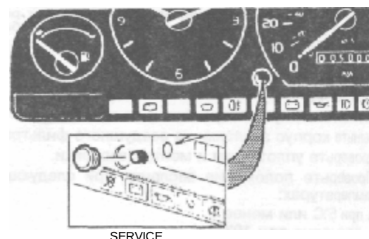
Рис. 4.8 Сброс индикатора обслуживания — исключая 240J-780 и 740 1990 г.
