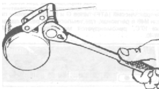
Рис. 1.22 Снятие масляного фильтра при помощи приспособления 2903
