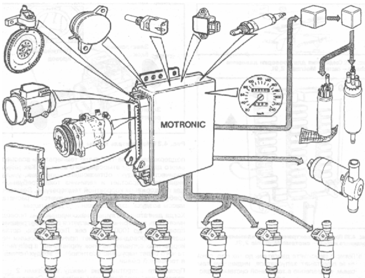
Рис. 4.28 Система впрыска топлива Motronic —двигатель B6304F объемом 2,9 л
