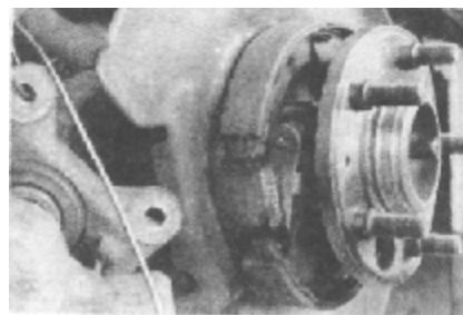
Рис. 9.23 Колодки стояночного тормоза — серия 940
