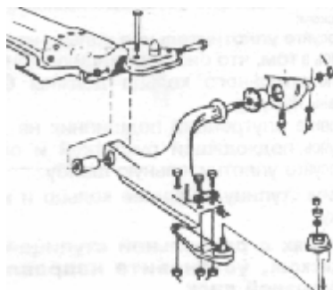
Рис. 8.6 Детали крепления нижнего рычага подвески — серия 240
