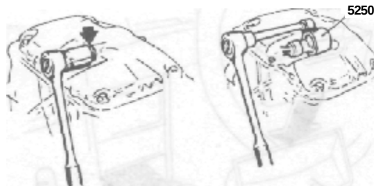
Рис. 7.3 Снятие выключателя фонаря заднего хода - A: коробка передач M46 и B: коробка передач M47
