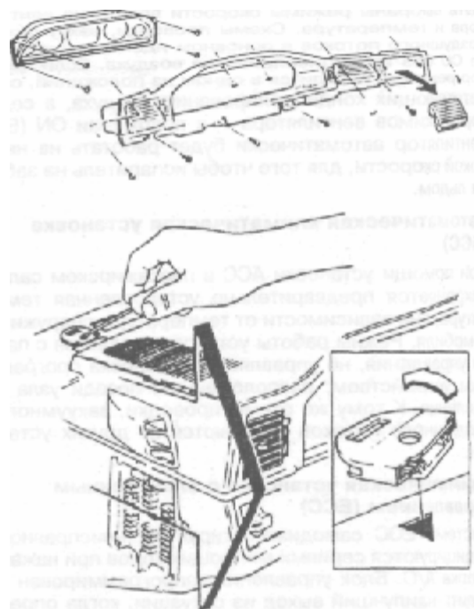
Рис. 6.16 Снятие приборной панели в сборе — 700 и 900 Серии
