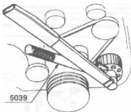
Рис. 3.45 Снятие приводного шкива масляного насоса при помощи упора — Двигатель B234F
