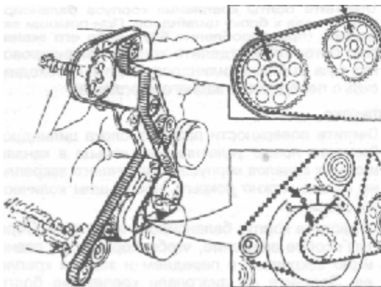
Рис. 3.67 Снятие приводного ремня и ремня балансировочных валов — Двигатель B234F
