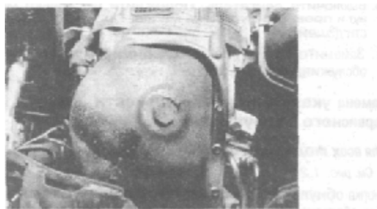
Рис. 1.20 Сливная пробка масляного поддона двигателя — показан B230FT
