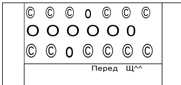
Рис. 3.32 Порядок затяжки болтов головки блока цилиндров — Двигатель B6304F
