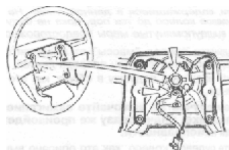
Рис. 8.24. Фиксация контактного кольца в нулевом положении
