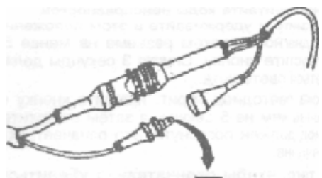
Рис. 5.26 Заземление провода датчика кислорода, идущего к блоку управления LH-Jetronic
