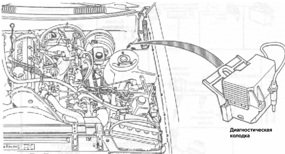
Рис. 4.17 Диагностическая тестовая колодка
