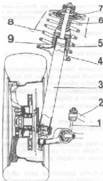
Рис. 8.5 Стойка с пружиной в сборе
