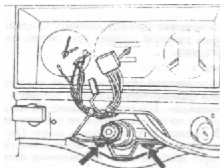
Рис. 8.27 Выбейте с помощью молотка срезающиеся болты из рулевой колонки
