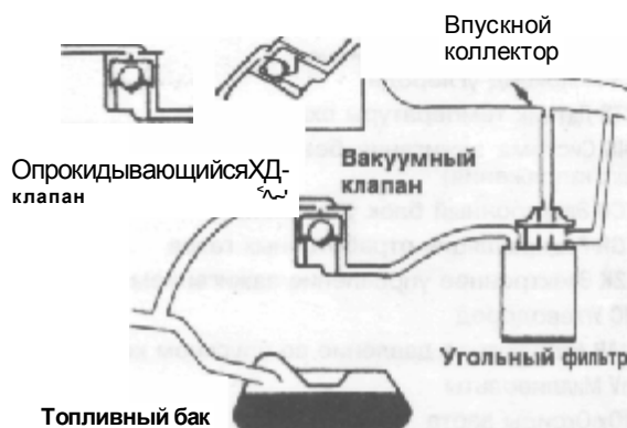
Рис. 4.4 Система EVAP — показано для 900-Серии
