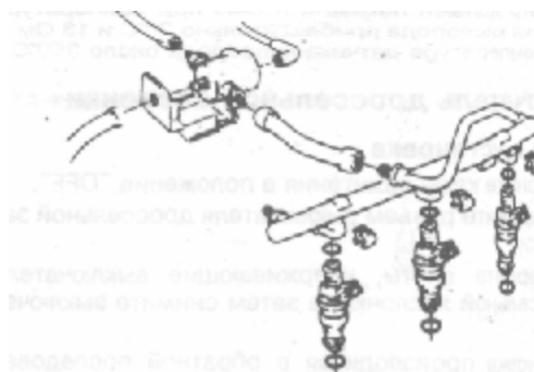
Рис. 5.13 Компоненты узла инжекторов в сборе двигатель B280F
