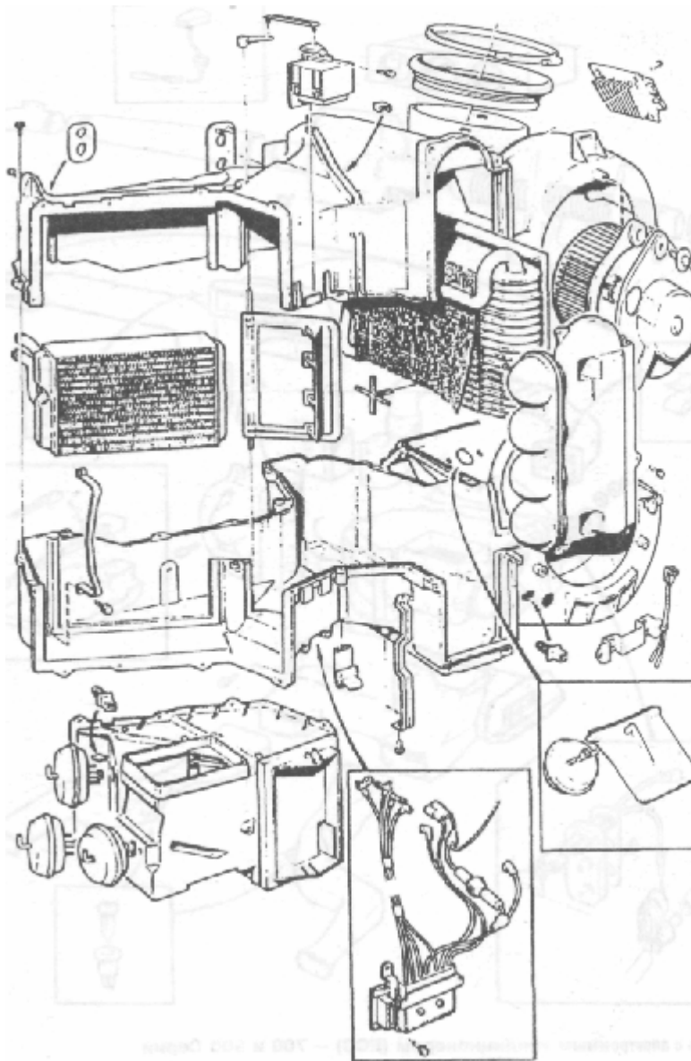
Рис. 6.12 Радиатор отопителя в сборе с электронным кондиционером (ЕСС) — 700 и 900 Серии
