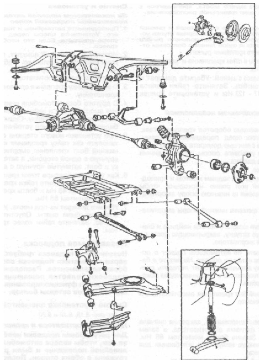
Рис. S.18 Элементы задней независимой подвески
