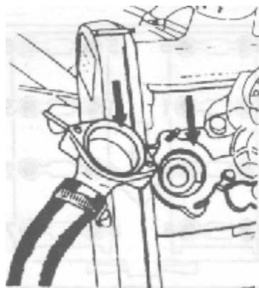
Рис. 3.18 Установка термостата в сборе — Двигатель B230F
