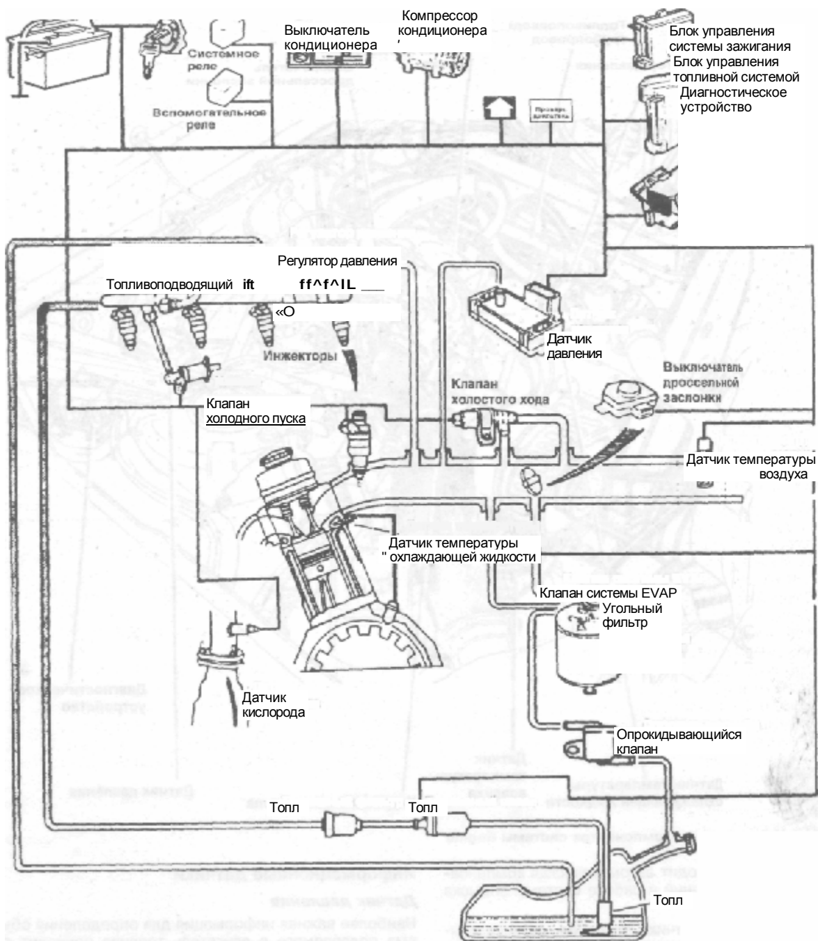
Рис. 5.42 Компоненты топливной системы Regina
