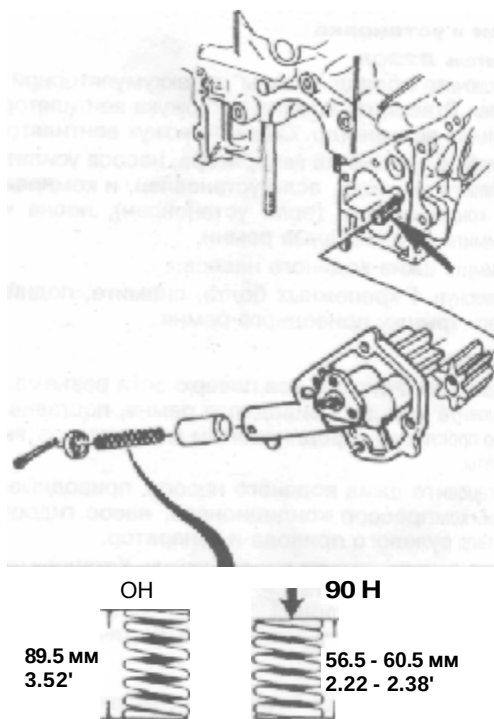
Рис. 3.50 Проверка деталей масляного насоса - Двигатель B280
