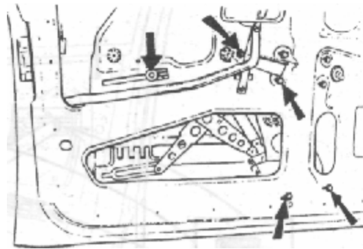
Рис. 10.17 Болты крепления привода стеклоподъемника — Серия 240
