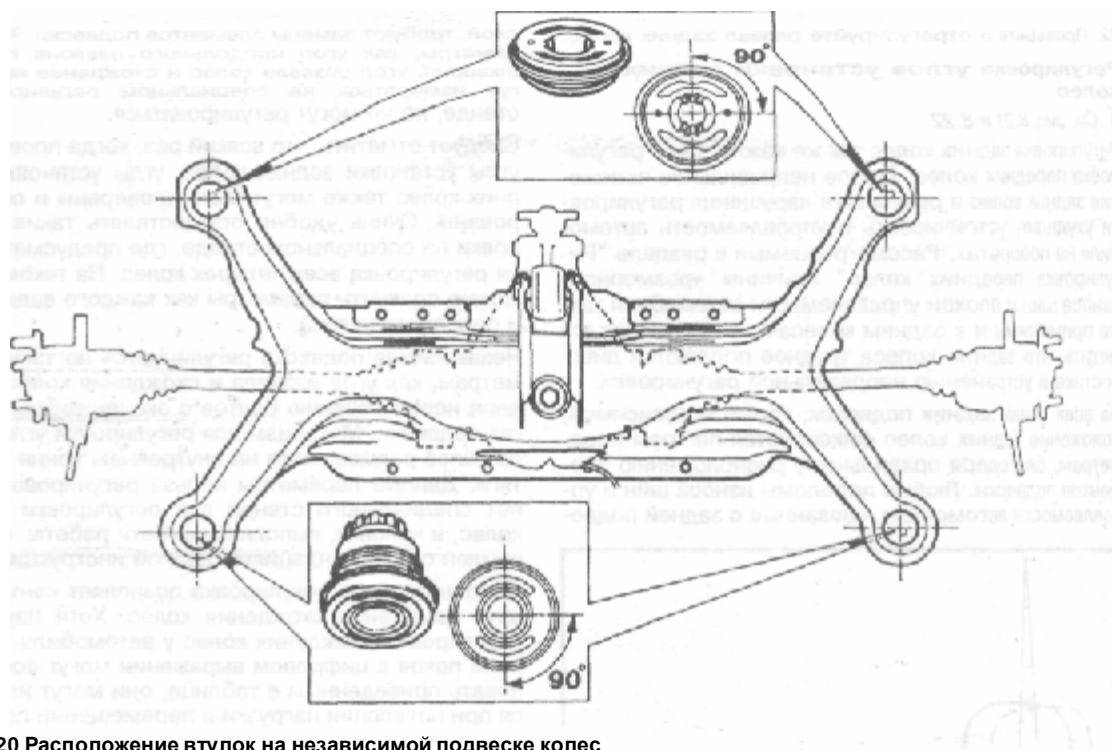
Рис. 8.20 Расположение втулок на независимой подвеске колес
