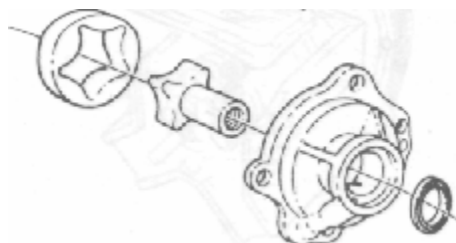
Рис. 3.48 Корпус масляного насоса и детали — Двигатель B234F
