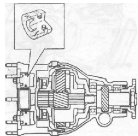
Рис. 7.5 Поперечный разрез узла повышающей передачи-коробка передач М46 с типами J или Р повышающей передачи
