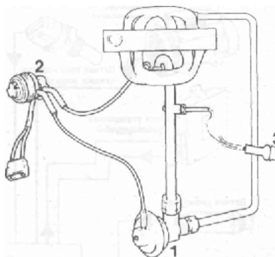
Рис. 4.41 Вакуум-схема работы системы EGR — двигатель B230F с системой зажигания 7E2K. 1. Вакуумный клапан EGR, 2. Вакуумный усилитель
