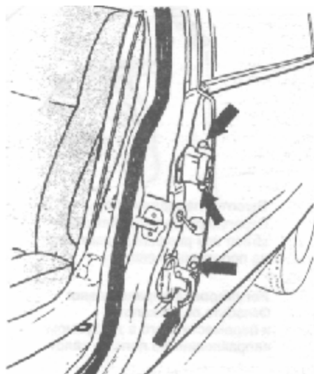
Рис. 10.3 Регулировка задней двери — Показана серия 700, на остальных — аналогично
