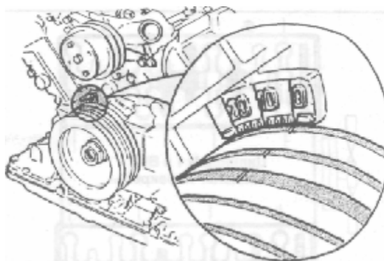
Рис. 2.51 При регулировке клапанов метка зажигания на шкиве должна совпадать с отметкой "О" на блоке двигателя — двигатель B280F
