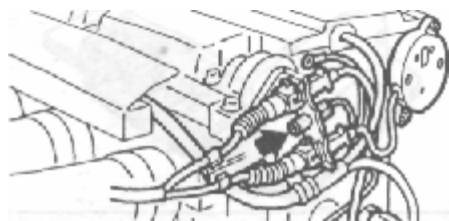
Рис. 5.101 Проверка напряжения на реле катушки зажигания — модель 960
