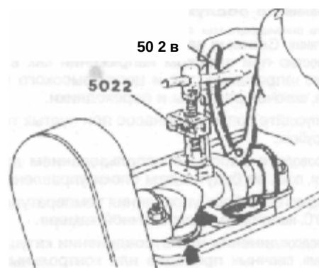
Рис. 2.47 Установка приспособления 5022 и удаление диска — двигатели B230F и B230FT
