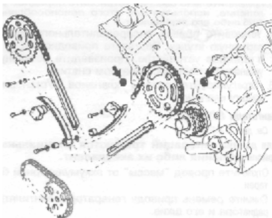
Рис. 3.60 Натяжное устройство цепи и цепь Двигатель B280F
