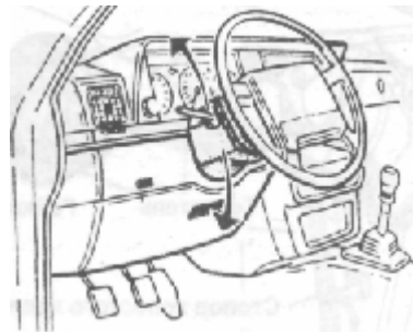
Рис. 6.23 Замена индикатора направления/переключателя круиз-контроля — показано для 240 серии
