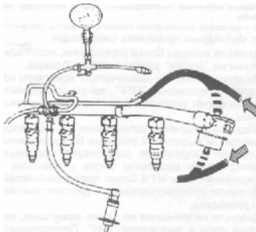
Рис. 5.19 Проверка шлангов регуляторов топлива — LH-Jetronic
