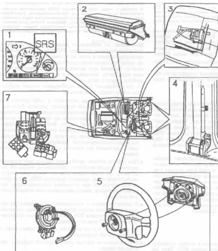
Рис. 6.1 Компоненты системы SRS
