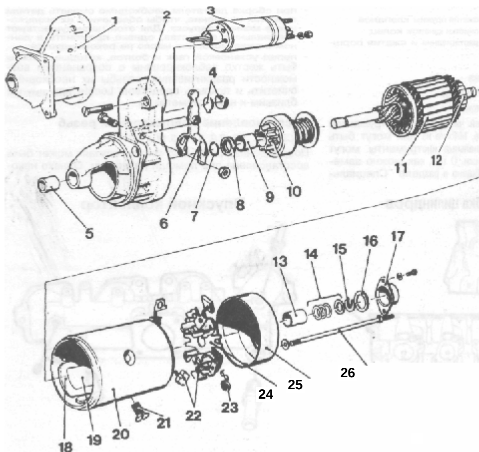
Рис. 3.7. Стартер Bosch
