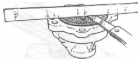
Рис. 3.47 Проверка осевого зазора роторов Двигатель B234F
